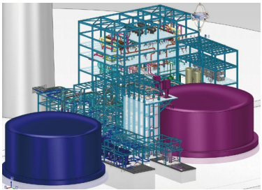
熔盐储换热系统三维图
