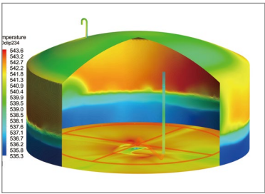
熔盐储罐进盐均流温度云图
